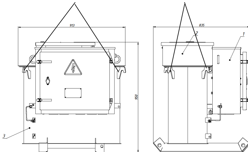
Рисунок А.1 - Габаритные размеры и масса КТПТО
